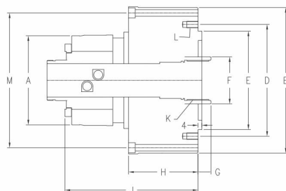
JAL中空氣壓迴轉缸
